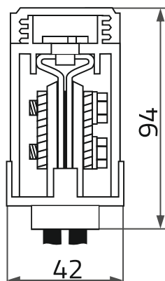
IZK-4-02 Izolacyjne złącza kablowe (fazowe). Cable joint
