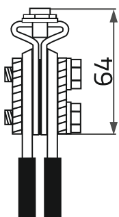
IZK-4-04 Izolacyjne złącza kablowe (zerowe nieizolowane). Cable joint (without isolation)
